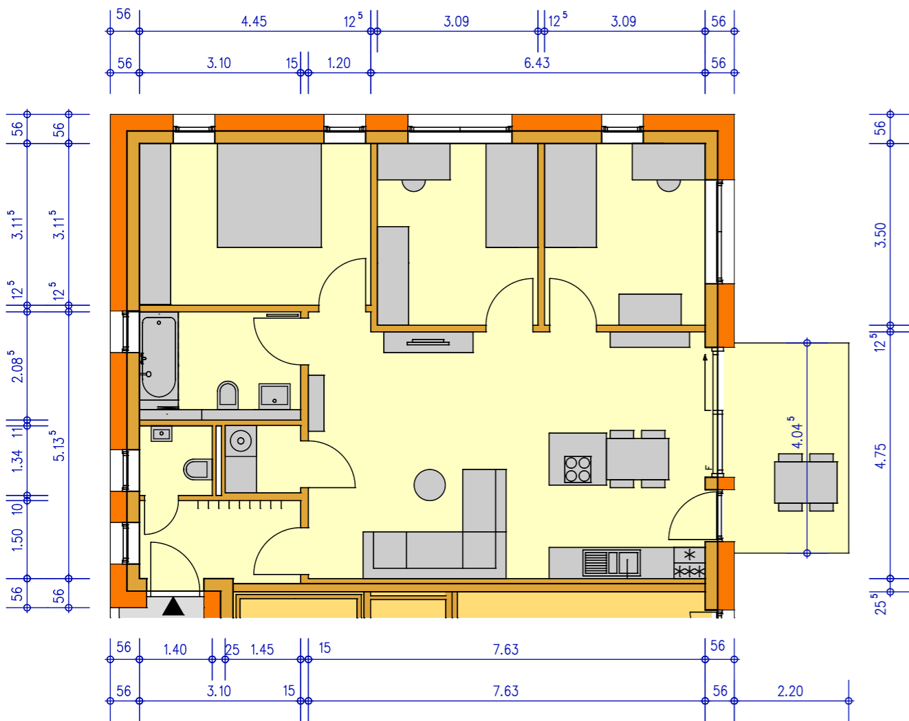
Grundriss M 1:100 (bei Ausdruck in DIN-A3)
